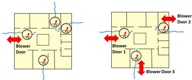
Abbildung 5: Gebäudegrundriss mit unterschiedlichen Möglichkeiten zur Messung der Druckdifferenz außen/innen:
